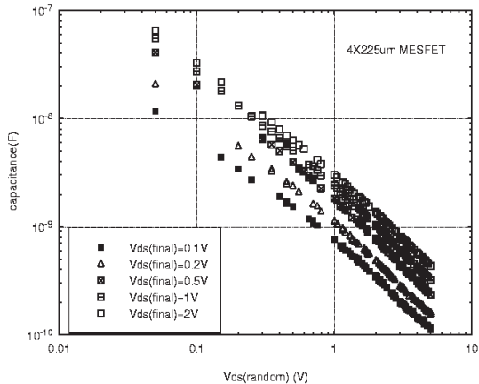
Figura 2: Capacidad obtenida de medidas pulsadas.
