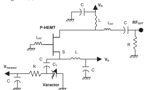
Fig. 1. Esquema eléctrico del oscilador controlado por tensión.
