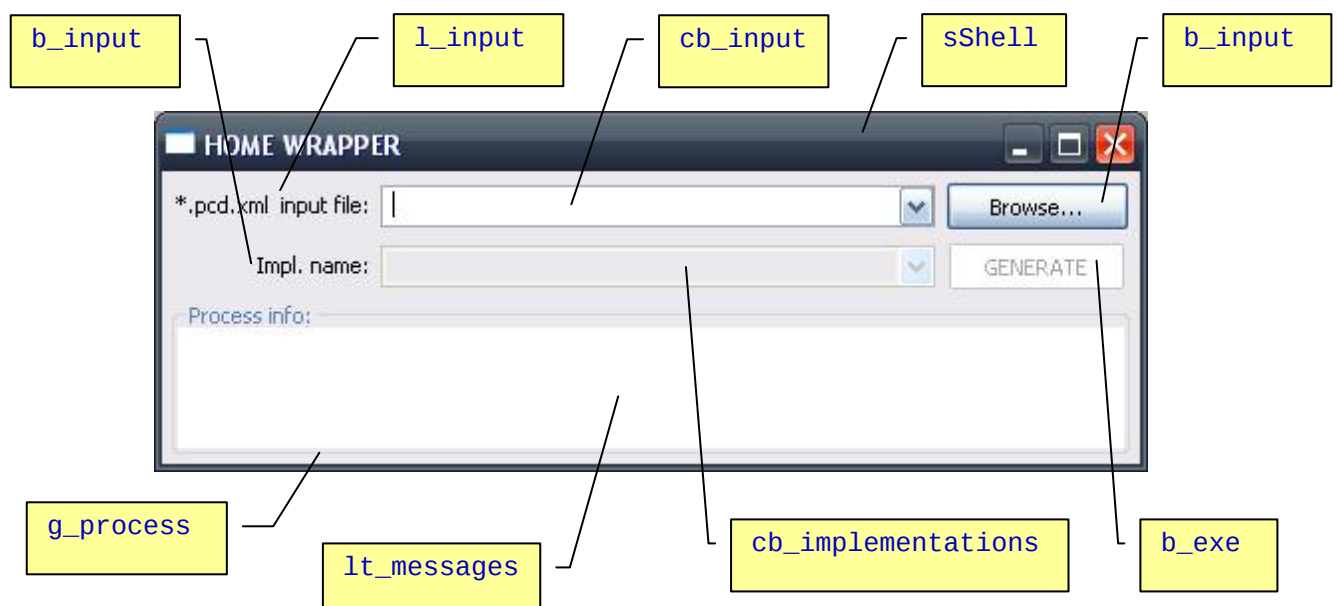
Figura 4.16 – Elementos GUI.
