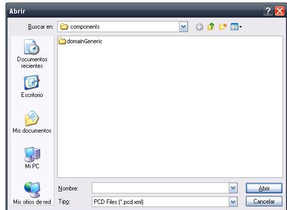
Figura 4.12 – Cuadro FileDialog .
