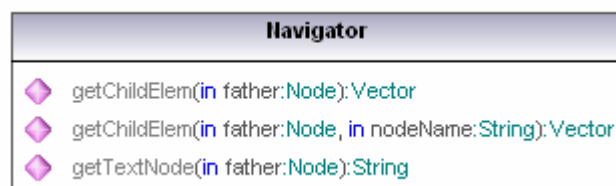
Figura 4.7– Clase Navigator .
