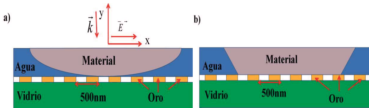
Figura 1.- Esquemas de las estructuras utilizadas para estudiar el efecto de un objeto de gran tamaño ( R=10\mu\text{m} ) sumergido dentro del agua. En a) la superficie de contacto entre el objeto y el array de nanoagujeros es mediante un punto. En b) el objeto cubre algunas nanorendijas con el fin de aumentar la superficie de contacto.
