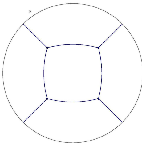
Triedro proyectivo
