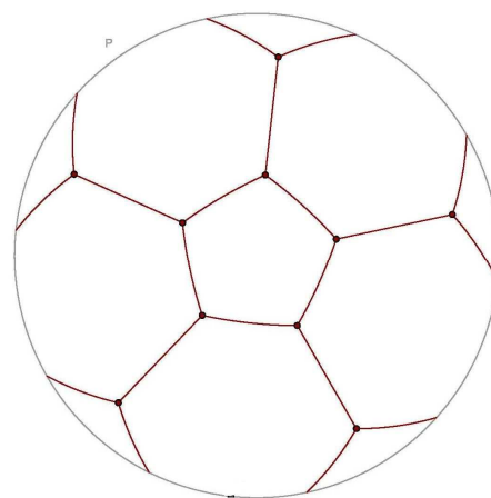
Hexaedro proyectivo
