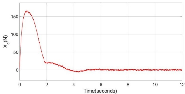
Figura 4 Resultados del ROV con L1 adaptativo; señal de control X_c(N) calculada por el controlador
