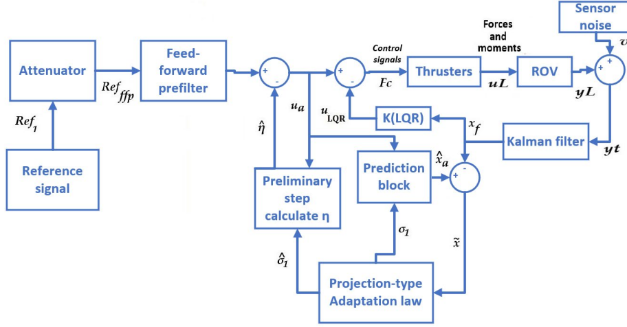
Figura 2 Esquema del sistema.
