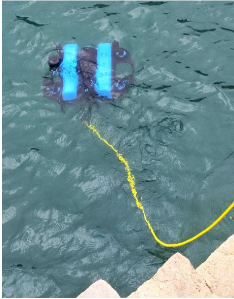
Figura 1 ROV de la casa Bluerobotics.
