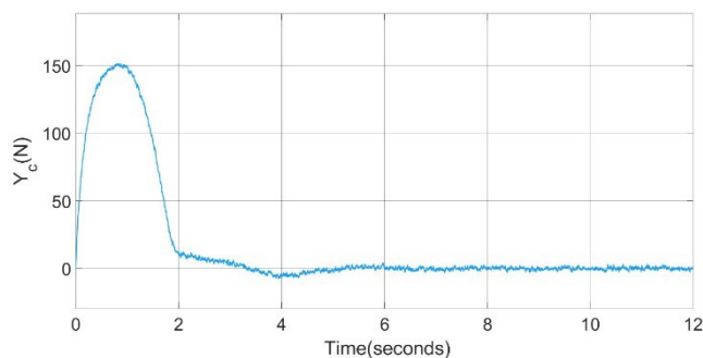
Figura 6 Resultados del ROV con L1 adaptativo; señal de control Y_c(N) calculada por el controlador
