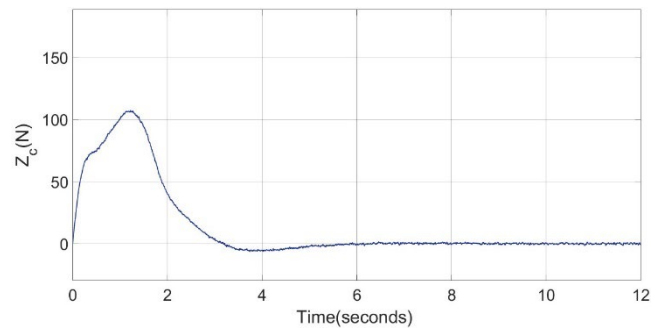
Figura 7 Resultados del ROV con L1 adaptativo; señal de control Z_c(N) calculada por el controlador.
