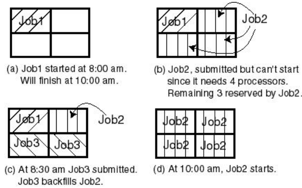
Figura 2.1: Algoritmo Backfilling 1
