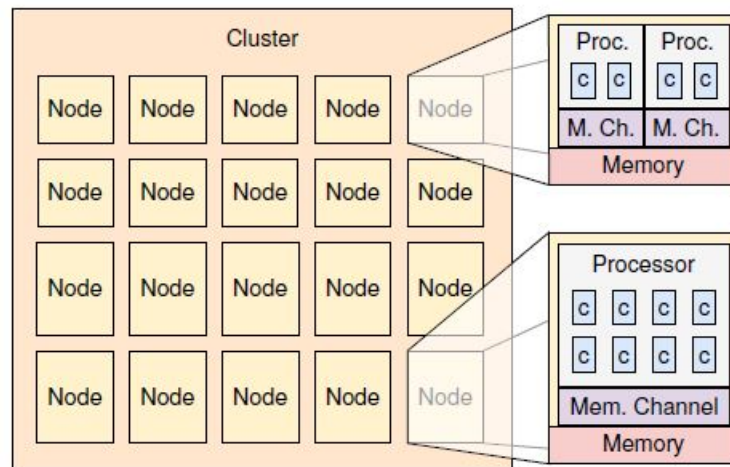
Figura 2.2: Cluster Heterogéneo 2
