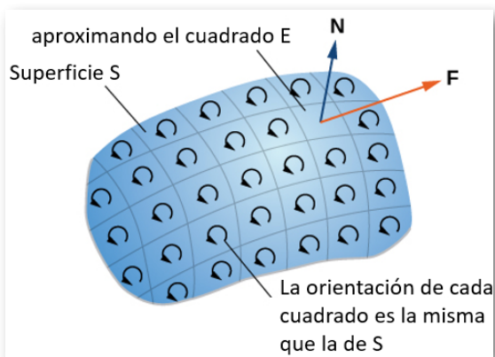
Figura 6.80. Pica la superficie en trozos pequeños. Las piezas deben ser lo suficientemente pequeñas como para que puedan aproximarse mediante un cuadrado.
