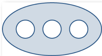
Figura 6.43. El teorema de Green, como se establece, no se aplica a una región no simplemente conectada con tres agujeros como este.
