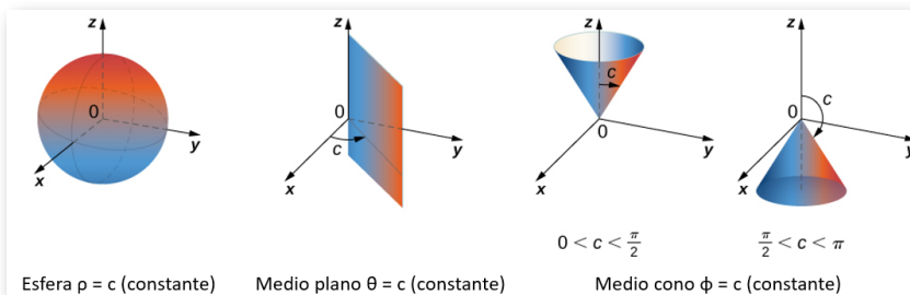
Figura 5.56. Las coordenadas esféricas son especialmente convenientes para trabajar con sólidos delimitados por este tipo de superficies (la letra c indica una constante).
