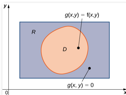
Figura 5.12. Para una región D que es un subconjunto de R , podemos definir una función g(x,y) para que sea igual a f(x,y) en cada punto de D y 0 en cada punto de R que no esté en D .
