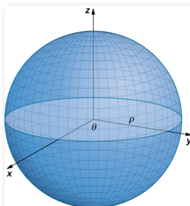
Figura 6.61. La esfera de radio \rho tiene parametrización \mathbf{r}(\phi, \theta) = \langle \rho \cos \theta \sin \phi, \rho \sin \theta \sin \phi, \rho \cos \phi \rangle , 0 \leq \theta \leq 2\pi , 0 \leq \phi \leq \pi .
