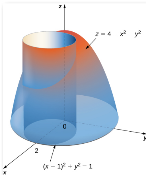
Figura 5.35. Encontrar el volumen de un sólido con una tapa paraboloide y una base circular.
