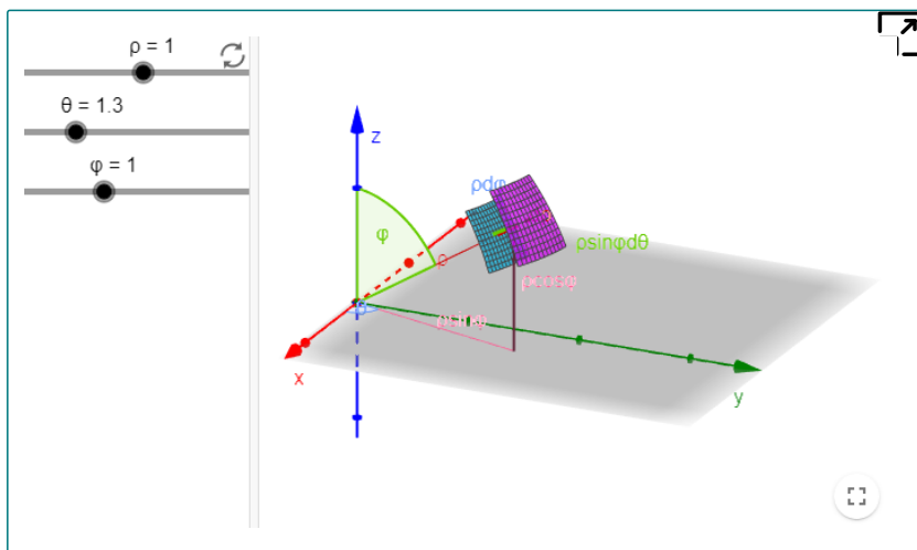
Figura 6.61. La esfera de radio \rho tiene parametrización \mathbf{r}(\phi, \theta) = \langle \rho \cos \theta \sin \phi, \rho \sin \theta \sin \phi, \rho \cos \phi \rangle , 0 \leq \theta \leq 2\pi , 0 \leq \phi \leq \pi .
