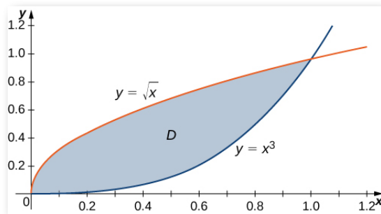
Figura 5.15. La región D se puede describir como Tipo I o Tipo II.
