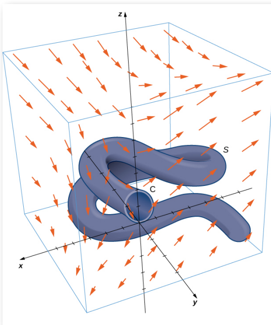
Figura 6.84. Una superficie complicada en un campo vectorial
