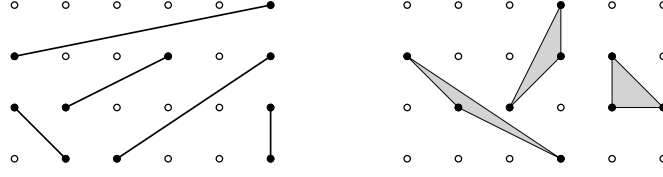
Figura I.3: La figura de la izquierda muestra segmentos reticulares unimodulares en el espacio ambiente \mathbb{R}^2 . Su volumen normalizado es uno en todos ellos, a pesar de que su volumen 2-dimensional es 0. La figura de la derecha muestra triángulos reticulares unimodulares.
